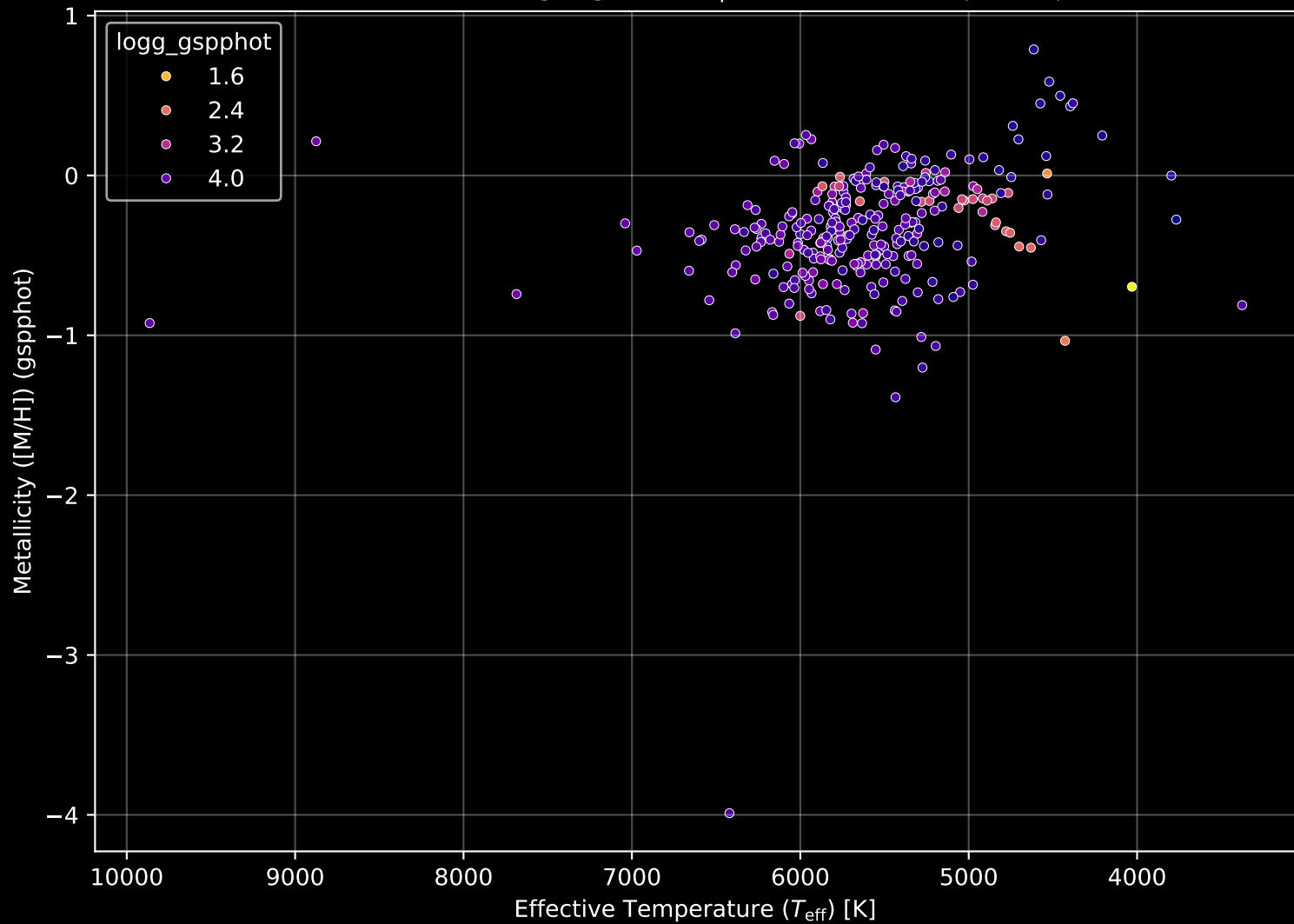
GALAH DR4 Field: [302] Stellar Population Parameters (n= 293)
