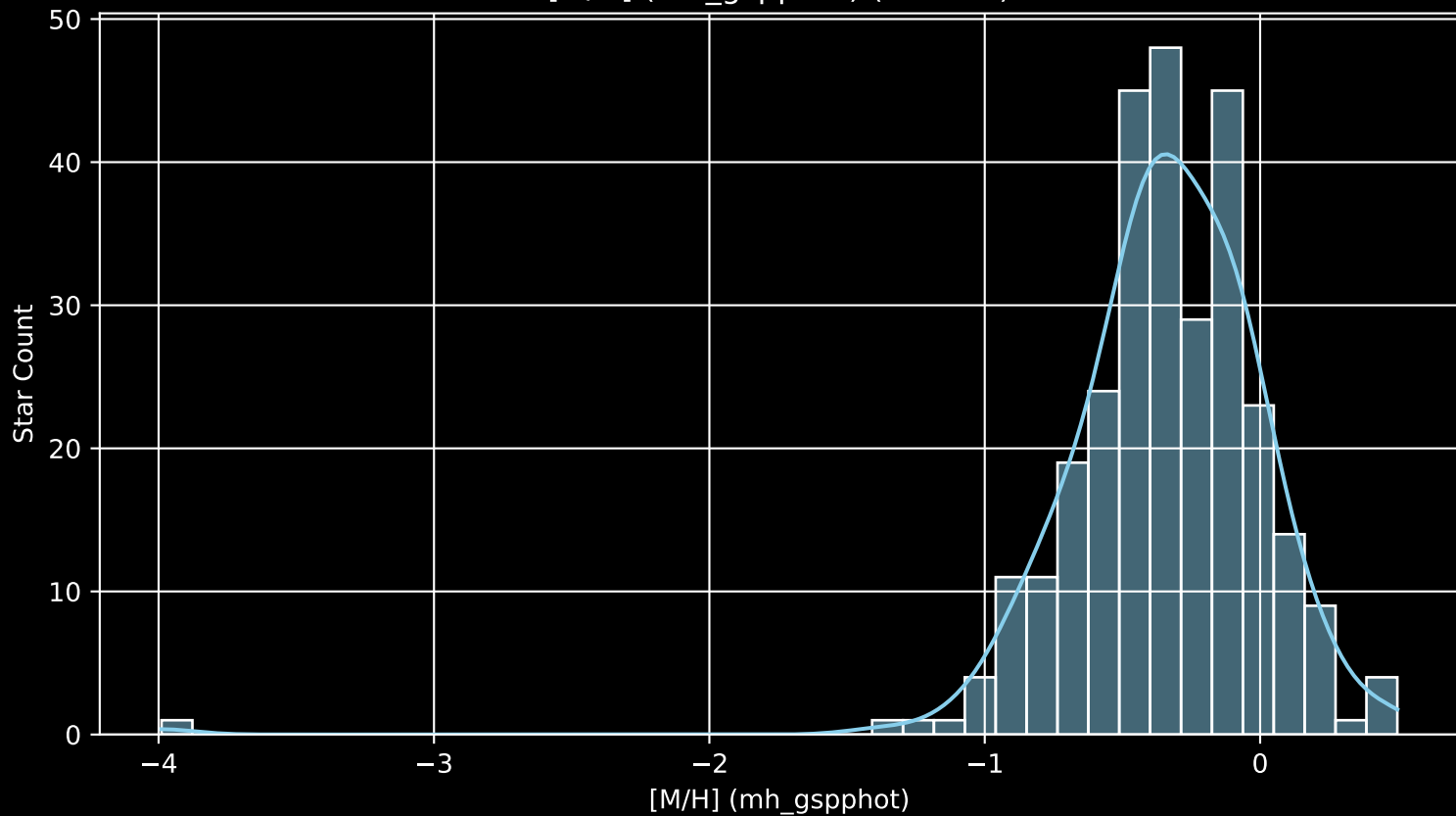
GALAH DR4 Field: [302] [M/H] (mh_gspphot) (n= 291)
